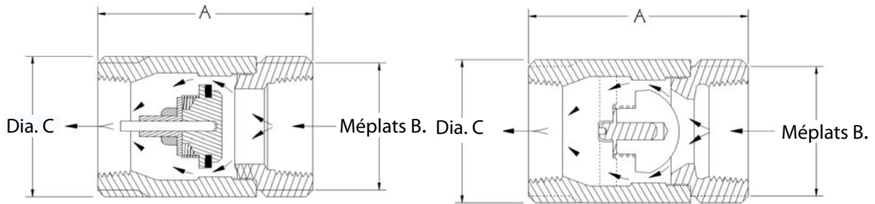
Clapets de 1/2" à 2"
